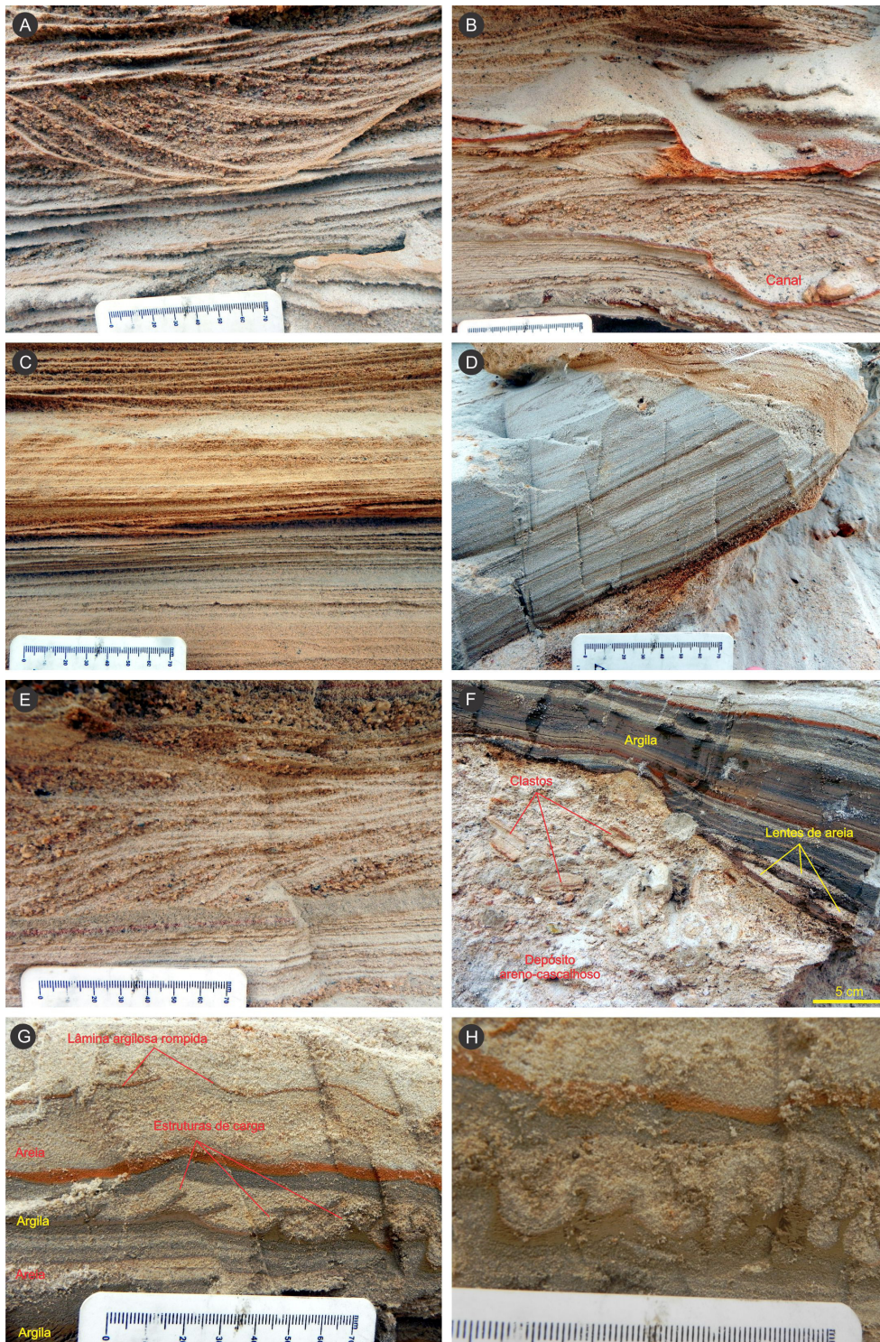
Figura 5. Produtos: Estruturas registradas em depósitos sedimentares no interior das lavras, visíveis em perfis transversais naturais ou artificiais. A) Depósito areno-cascalhoso preenchendo canal, com laminação marcando a migração do canal para a direita da imagem; B) Canal preenchido por sedimento cascalho-arenoso, recoberto por depósito arenoso com laminação plano-paralela e cruzada; C) Laminação plano-paralela; D) Laminação transladante em depósito arenoso eólico; E) Laminação cruzada sigmoidal, registrando o avanço de um pequeno delta arenoso sobre substrato silto arenoso horizontal; F) Depósito areno-cascalhoso recoberto por depósito argilo-arenoso laminado, exibindo lentes de areia; G) Camadas de argila intercaladas em depósito arenoso, exibindo estruturas de carga e lâminas argilosas rompidas; H) Detalhe das estruturas de carga.
