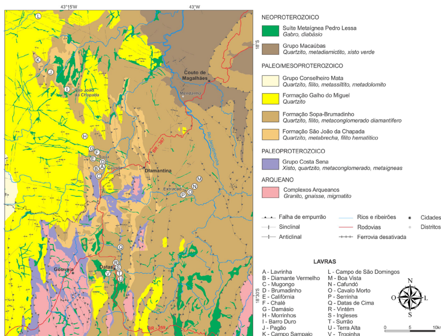
Figura 1. Mapa geológico simplificado da região de Diamantina, modificado de Fogaça (1996), Tupinambá et al. (1996), Knauer & Grossi Sad (1996), Knauer & Fogaça (1996), Noce & Fogaça (1996) e Roque et al. (1996). Destaque para a localização das principais lavras de diamante da região, atualmente desativadas.
