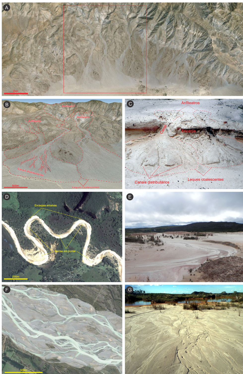
Figura 7. Exemplos de análise escalar a partir das feições observadas nas lavras da região de Diamantina. A) Imagem de satélite das Montanhas Santa Rosa, USA, mostrando o desenvolvimento de um complexo sistema de leques aluvionares; B) Detalhe dos leques observados na figura anterior, com destaque para os elementos morfológicos dos leques; C) Leques observados no interior de uma lava, para comparação; D) Imagem de satélite mostrando o Ribeirão de Areia, curso d'água meandrante de Chapada Gaúcha (MG), com destaque para seus elementos morfológicos; E) Meandro observado no interior da lava, para comparação; F) Imagem de satélite exibindo trecho entrelaçado do Rio Waimakariri, Nova Zelândia; G) Curso d'água meandrante observado no interior da lava, para comparação.
