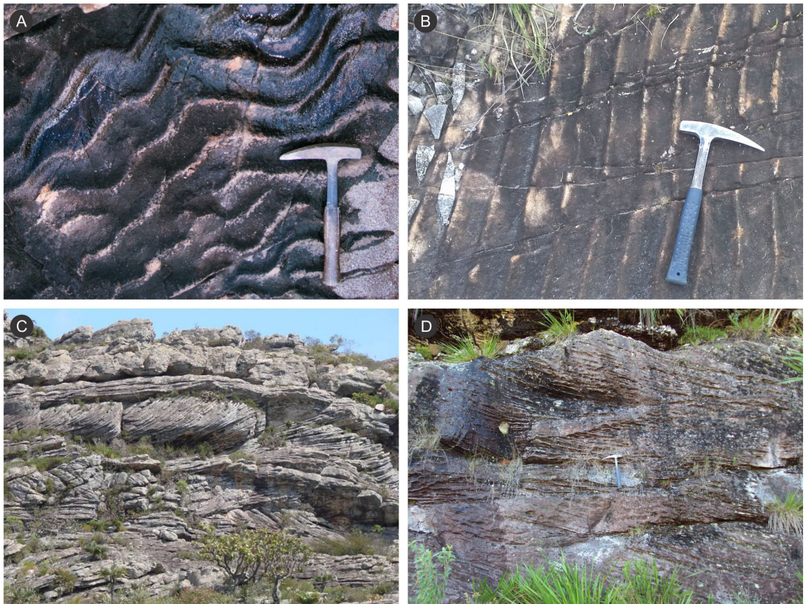
Figura 8. Estruturas sedimentares em quartzitos do Supergrupo Espinhaço na região de Diamantina. A) Ripples assimétricas de crista sinuosa; B) Ripples assimétricas de crista reta; C) Estratificação cruzada tangencial à base, de porte métrico; D) Estratificações cruzadas acanaladas.
