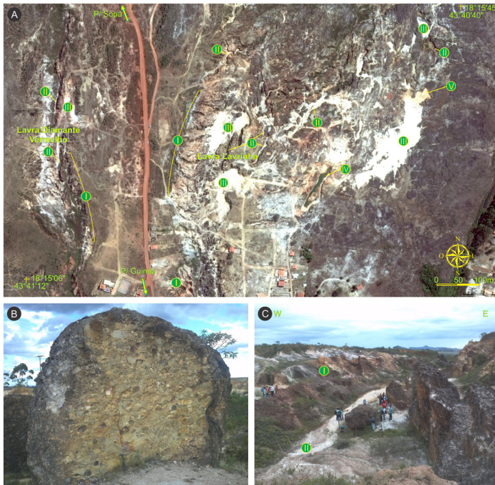
Figura 2. Aspecto geral das lavras desativadas da região de Diamantina (MG). A) Imagem de Satélite (Google Earth®) da região a norte de Guinda, distrito de Diamantina, exibindo duas das principais lavras da região: Lavrinha e Diamante Vermelho. Notar o relevo extremamente irregular no interior da lava, e a ocorrência das seguintes feições, indicadas por números: I – Feições erosivas, II – Canais, III – Sítios de deposição, IV – Corpo d’água perene, V – Corpo d’água sazonal. B) Afloramento de metaconglomerado polimítico da Formação Sopa-Brumadinho no interior da Lavra Lavrinha. O afloramento foi preservado da atividade de lava por apresentar-se extremamente silicificado, enquanto as porções adjacentes, mais friáveis, foram lavradas. C) Interior da Lavra Diamante Vermelho, com destaque para a extrema irregularidade do relevo.
