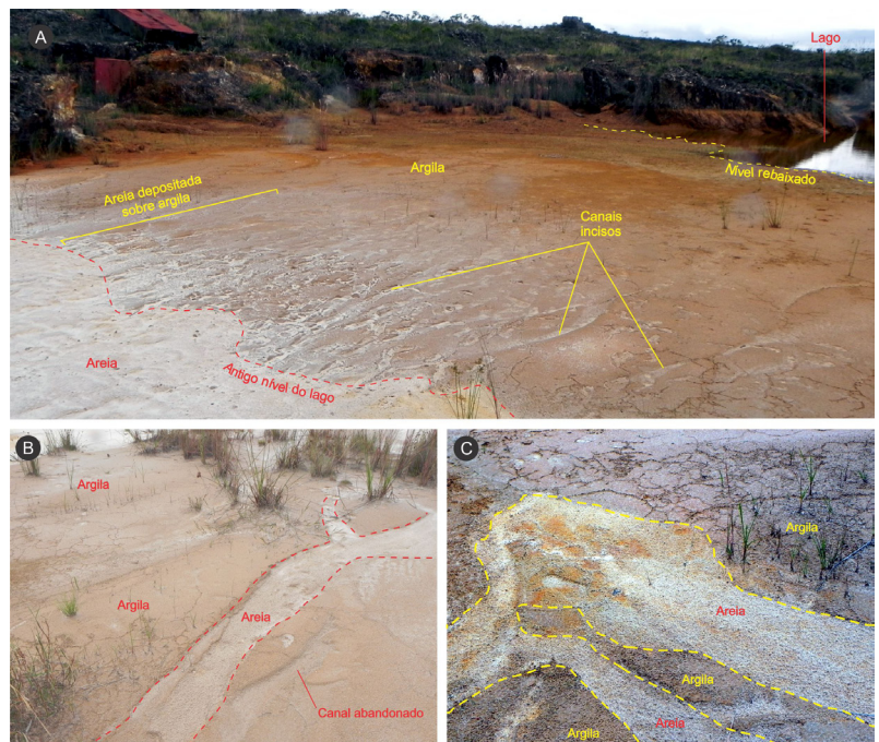
Figura 4. Dinâmica de processos sedimentares no interior da lavra, em resposta ao rebaixamento sazonal do nível de base local. A) Deposição de areia por processos eólicos e fluviais sobre os depósitos argilosos lacustres; B) Detalhe de pequenos deltas arenosos coalescentes, formados na extremidade de canais incisos nos depósitos argilosos lacustres.
