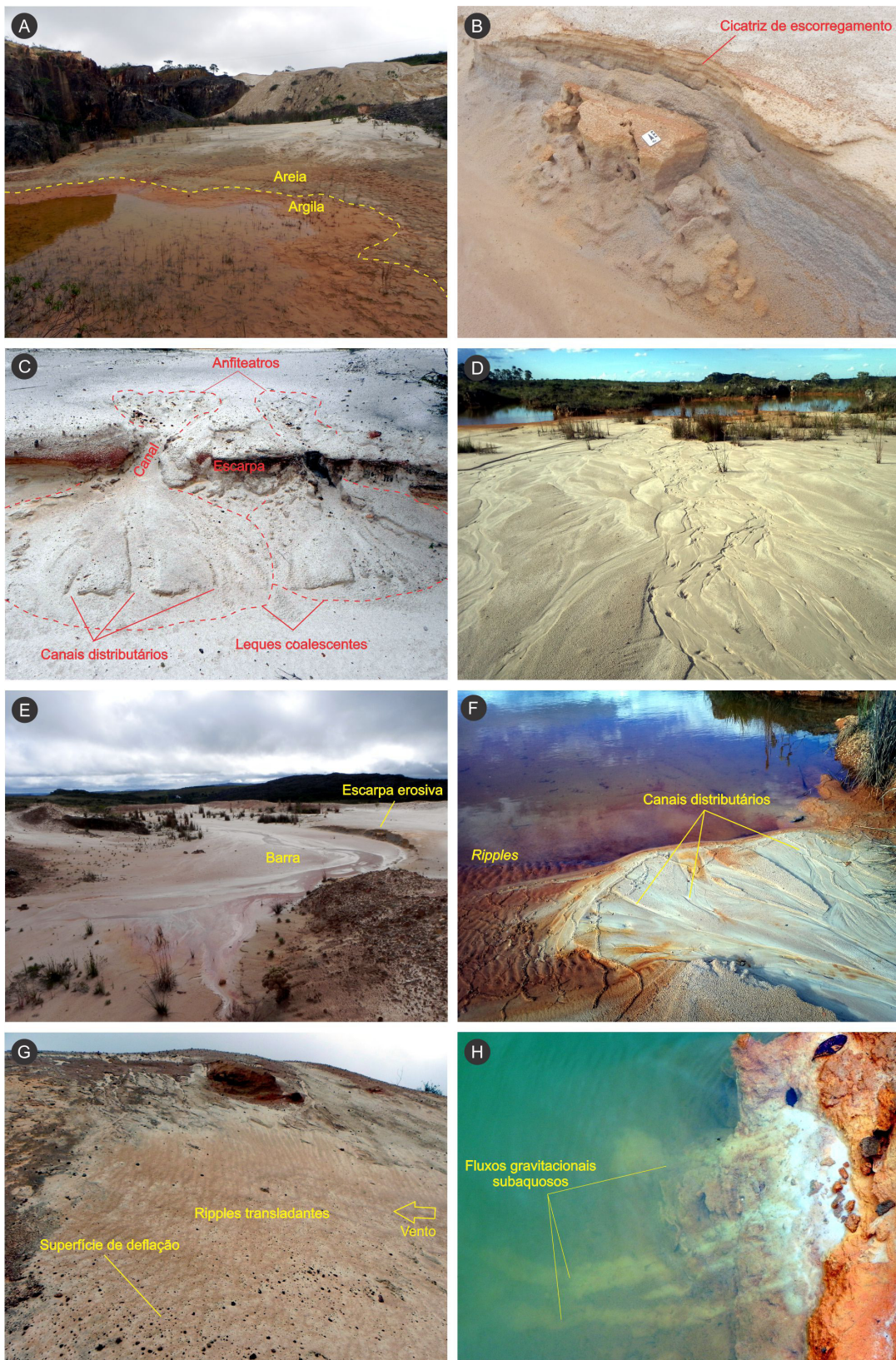
Figura 3. Processos sedimentares observados em diferentes ambientes de sedimentação no interior de lavras desativadas na região de Diamantina (MG). Ver texto para detalhes. A) Lacustres; B) Movimentos de massa; C) Leques aluviais; D e E) Fluviais; F) Deltaicos; G) Eólicos; H) Fluxos gravitacionais subaquosos.
